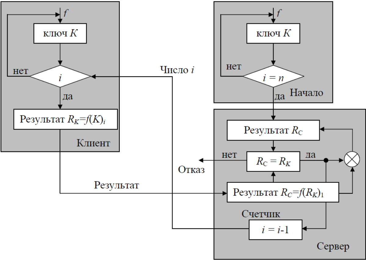
Рисунок 1.9 – Программный генератор одноразовых паролей S/KEY
